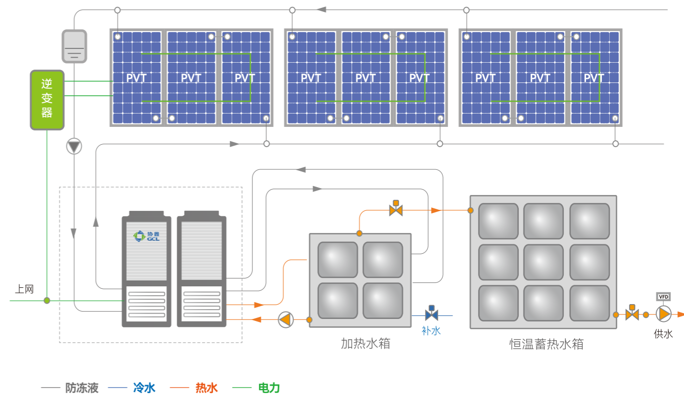
▶ PVT双源热泵热水系统示意图
